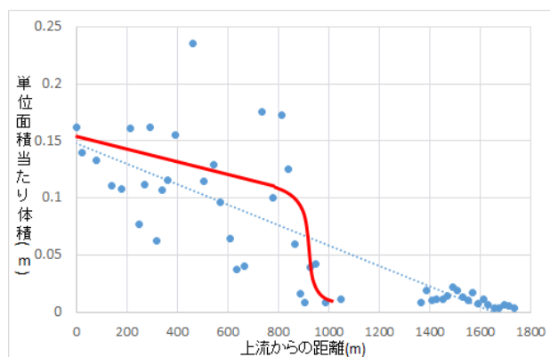
図-8 ダム上流部における流木の縦断分布
