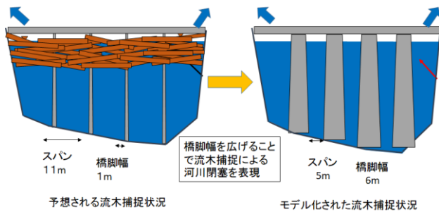
図-10 モデルにおける流木集積の設定
