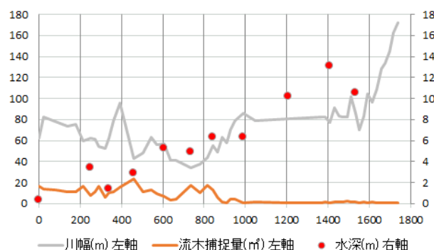
図-9 川幅, 水深と流木量の関係
