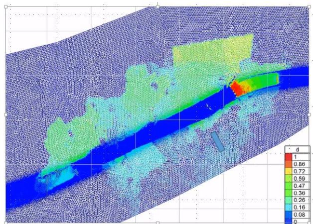
図-13 尾形原橋における流木集積有無による氾濫水深差
