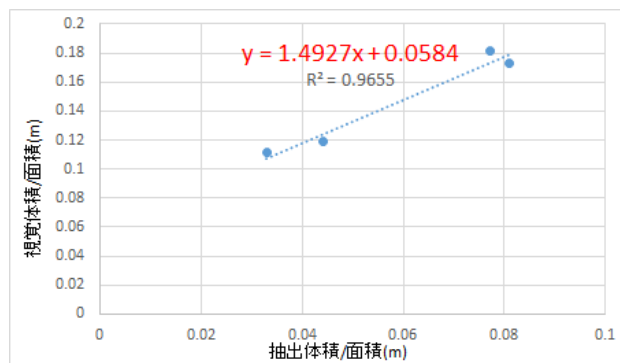
図-4 上流側の流木量推定の補正式
