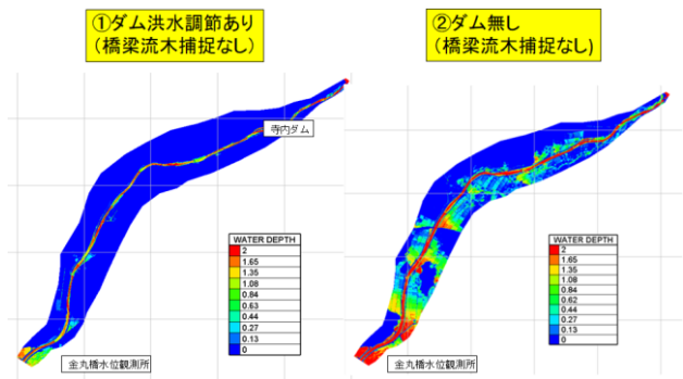
図-11 洪水調節ありとなしの計算結果
