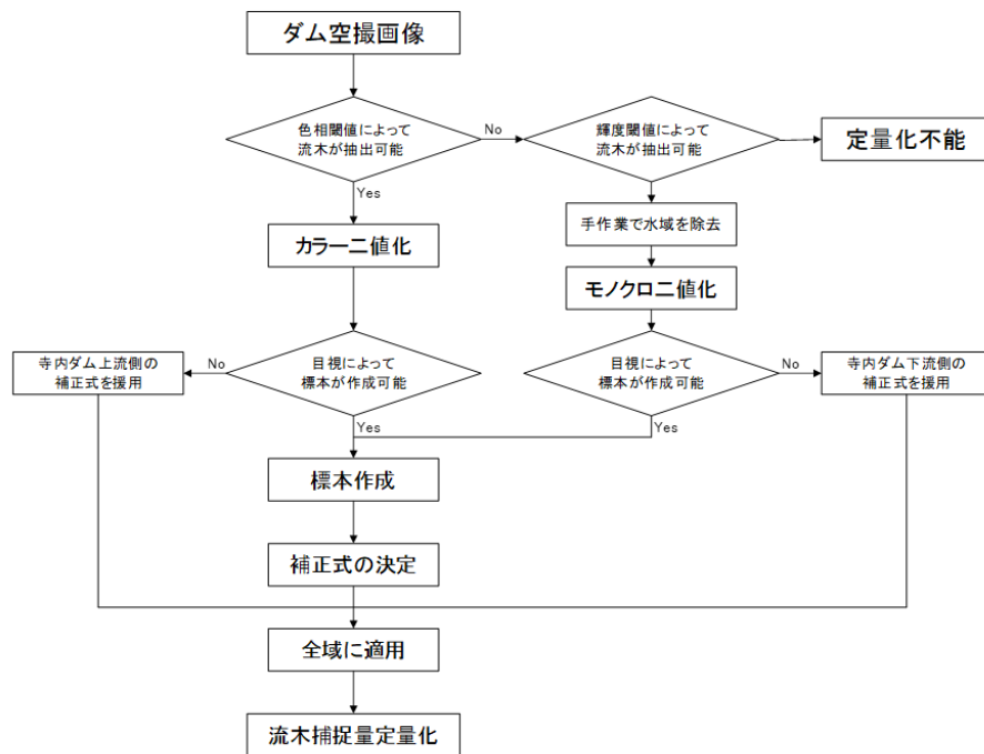
図-5 画像からの流木抽出と流木量推定のフローチャート
