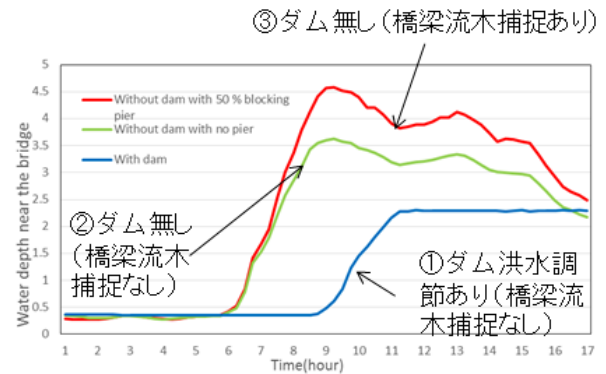
図-12 尾形原橋における水位の変化
