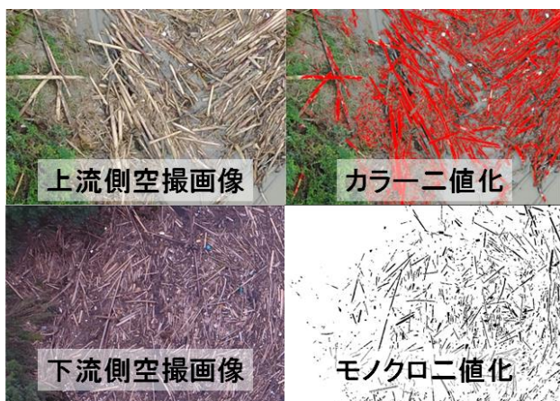
図-2 寺内ダムにおける流木の集積状況（上：集積範囲，下左：貯水池下流，下右：貯水池上流）
