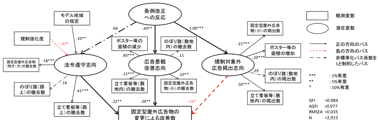
図-6 共分散構造分析の結果 (標準化解)
