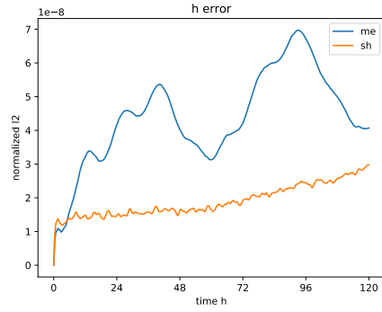
図4 Case 2 (a), 3(b) における高度の規格化された \ell_2 ノルム。青及び橙はそれぞれ最小エネルギー及び球面螺旋節点を表す。
