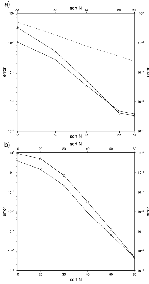
図3 (a) cos 型 ( N = 529, 1024, 1849, 3136, 4096 , 破線は N^{-3/2} ), (b) ガウス型の山 ( N = 100, 400, 900, 1600, 2500, 3600 ) の移流実験。○ 及び × はそれぞれ \ell_2 及び \ell_{\text{inf}} ノルム。
