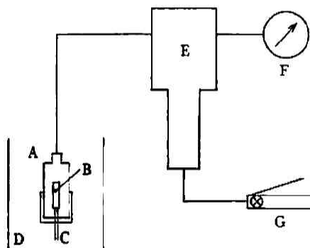
Fig. 1 Apparatus
