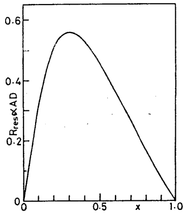
第1図 残留抵抗 ( R_{\text{res}} \propto AD ) の x 依存性
