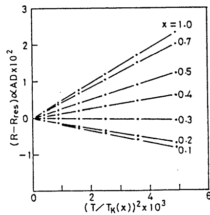
第3図 低温の電気抵抗 ( R - R_{\text{res}} \propto AD ) の T^2 依存性
