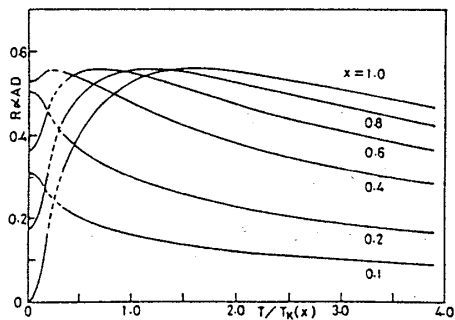
第4図 電気抵抗の温度変化
