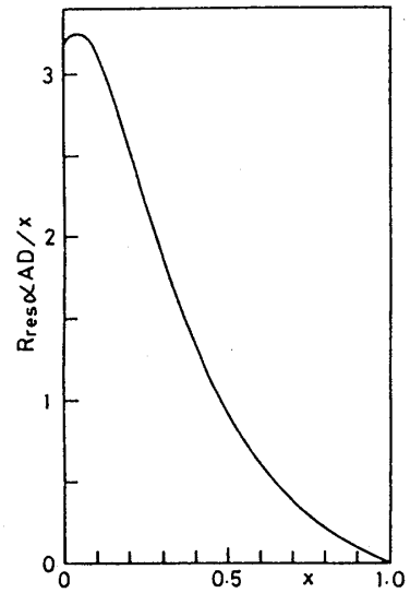
第2図 R_{\text{res}} \propto AD / x の x 依存性
