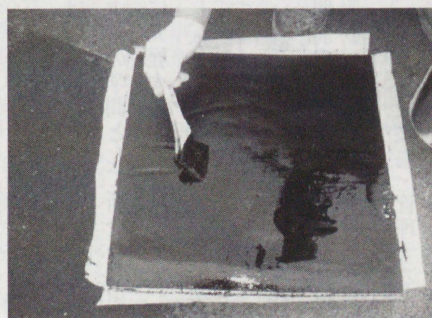
写真2 専用接着剤の塗布
