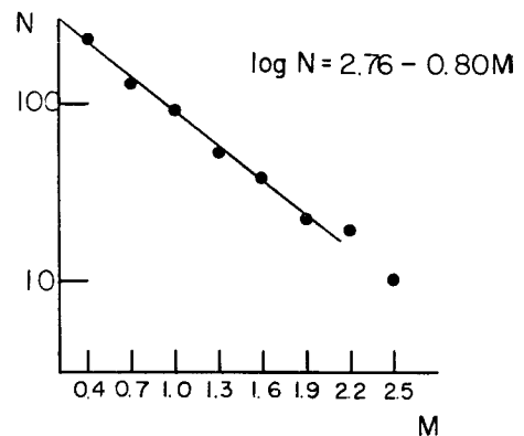
Fig. 7 Gutenberg-Richter' relation.
