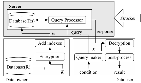
図 1: 暗号化データベースモデルにおける 4 プレーヤ．
