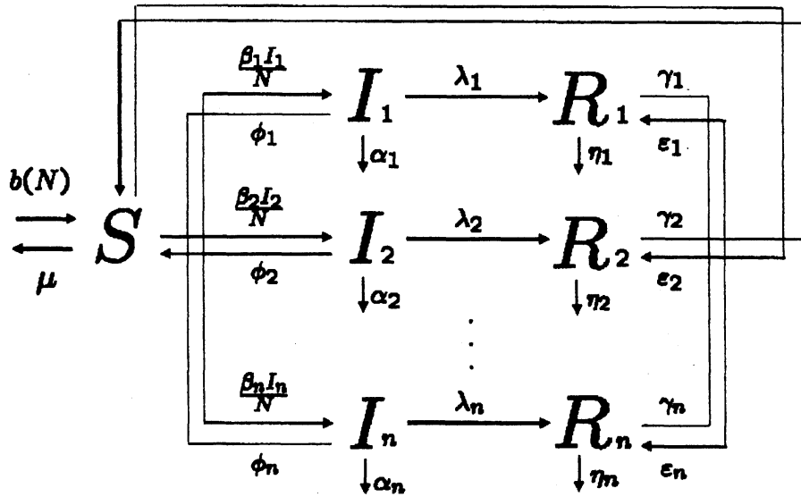
図 2: N 種の毒性をもつ伝染病モデルのダイアグラム
