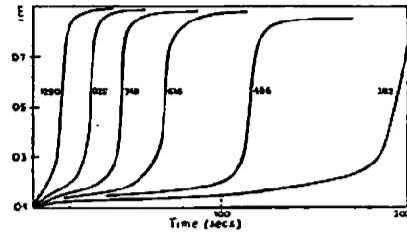
第六圖 0.05%キノヒドロン溶液の陰極還元に於ける電壓時間曲線 (数字は 4.3 cm 2 電極に對する電流の強さ (amp × 10 -6 ))
