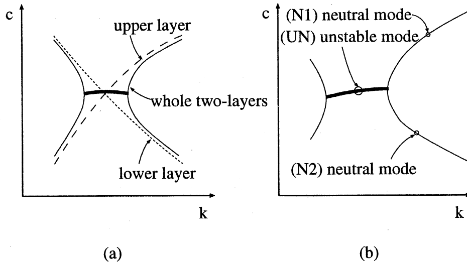
図 3: 共鳴による不安定モードの理解。(a) 2層問題のように部分系が構成できる場合。2層問題全体を解いた時の不安定モードは上層1層問題と下層1層問題の分散曲線の交点にある。(b) 部分系が容易には構成できない場合。不安定モードにつながる二つの中立モード (N1), (N2) の構造を調べることによって、不安定モード (UN) がどのようなモードの共鳴で起きたかわかる。
