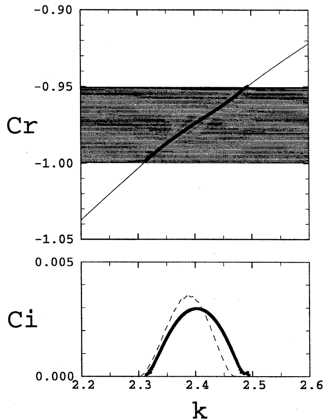
図 4: 基本流速を差し引いた正則モードの位相速度が負、下層の渦位勾配が負の時に起こる臨界層不安定の分散関係。下層の基本流速の範囲 -1.00 \sim -0.95 には、離散化された連続モードが見られる。
