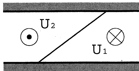
図 1: Iga (1993) で安定性を解析した前線のモデル
