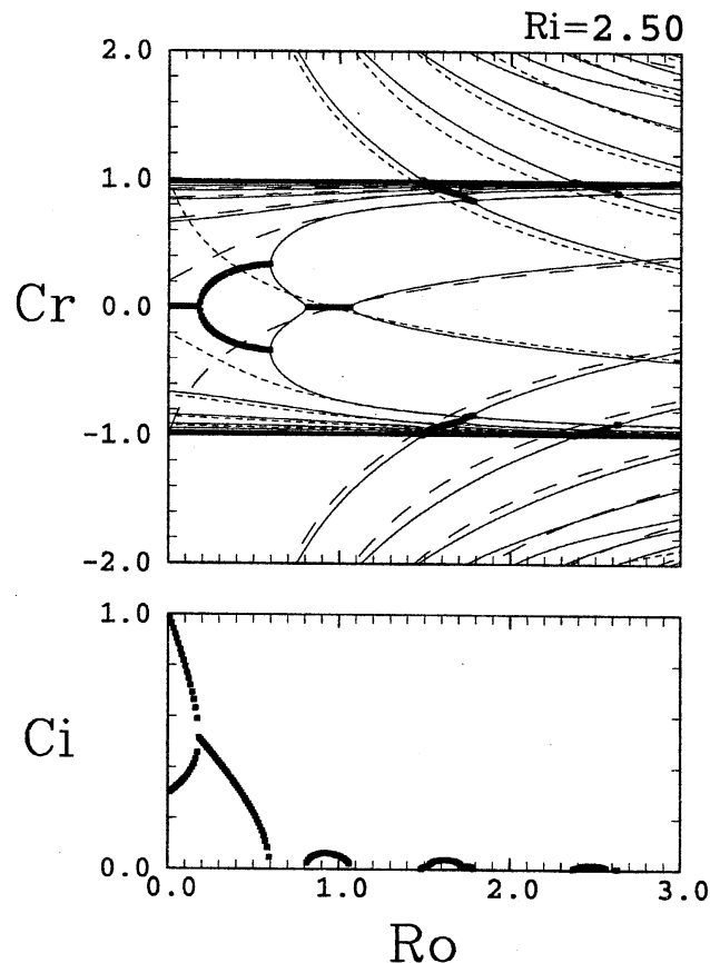
図 2: Ri (基本場を特徴づける無次元パラメータ) が 2.5 の時の前線不安定問題の分散関係 (実線)。太線は不安定を表す。破線は上層 1 層問題、点線は下層 1 層問題の中立波の分散曲線。
