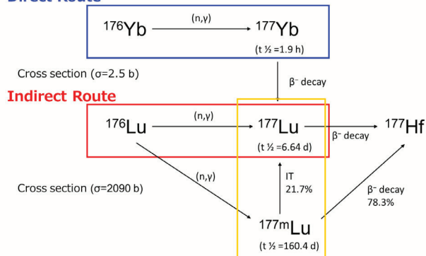
Fig. 1. 177 Lu Production Process
