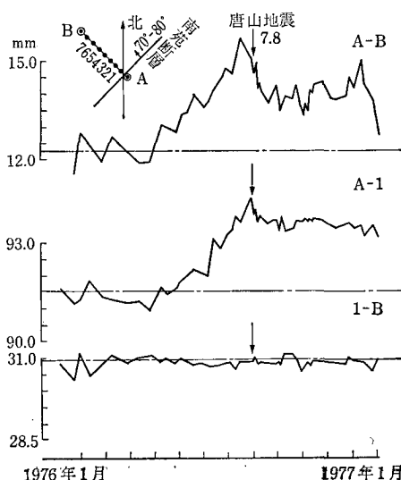
図47 範庄子短水準の上下変動のデータ
