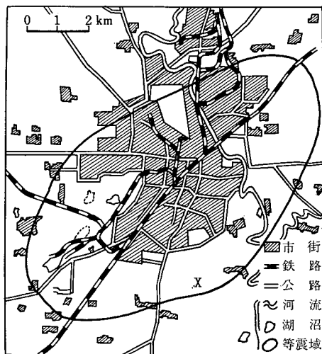
図16 唐山地震の震度分布
