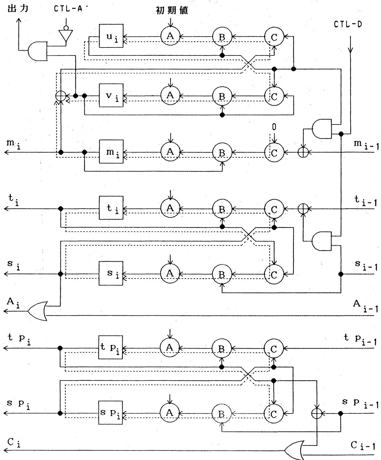
(図8-d) フェイズ4のデータの流れ
