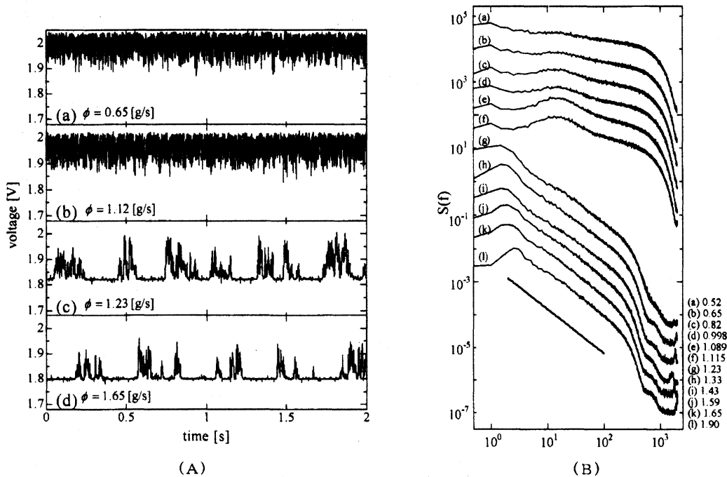
図5 : (A) パイプの上端から 80cm の位置で測定した、粉粒体の流入量 \phi (g/s) を変えたときのレーザー透過強度の時系列。(B) レーザー透過強度の時系列に基づいて得られたパワースペクトル。図の右下にある (a) ~ (l) の値は、粉粒体の流入量 (g/s) を表しており、図中にプロットされた曲線の左上にある (a) ~ (l) と対応している。図中の直線は、べき指数が 4/3 を示すガイドラインである。
