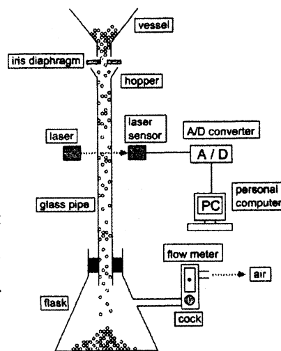
図1：実験装置の模式図。
