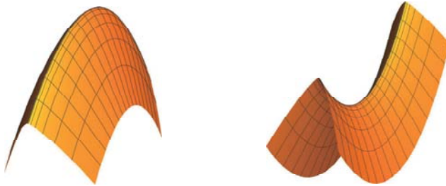
図3 左: \Pi_{3,4} > 0 のカスプ辺, 右: \Pi_{3,4} < 0 のカスプ辺.
