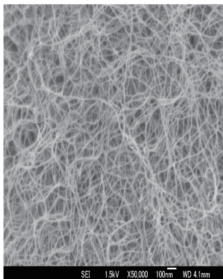
図1 木材細胞壁中のセルロースナノファイバー。図中のバーは100nm。
