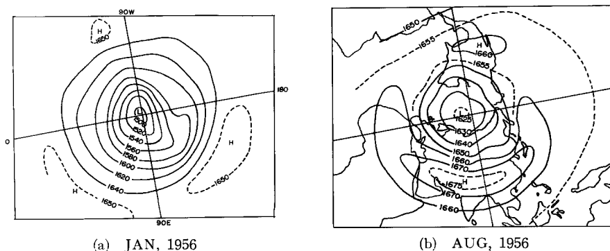
Fig. 1 100 mb 天 気 図
