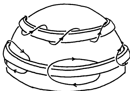
Fig. 2 プラネタリー波と中緯度高圧帯中の空気の軌道モデル
