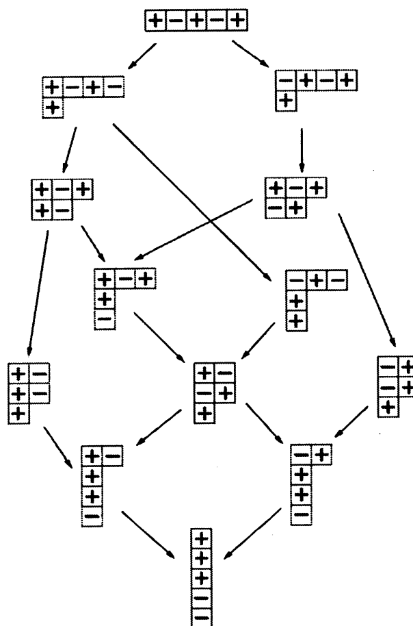
FIGURE 1. U(3, 2) の巾零 K 軌道と閉包関係
