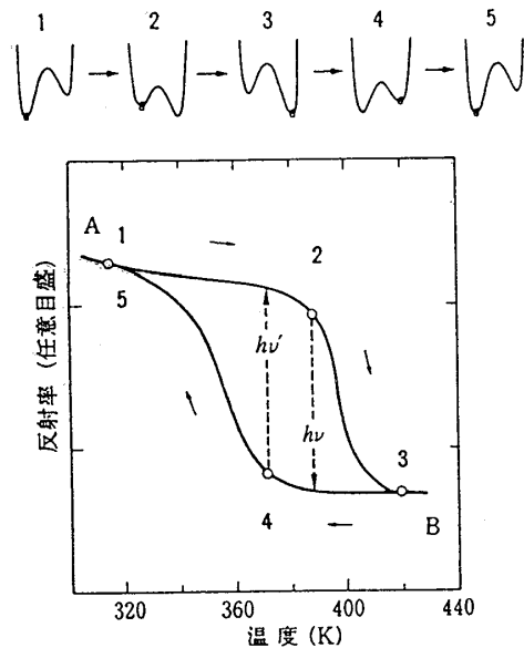
第8図 Poly-4U3単結晶の1.95 eVにおける反射率の温度変化。ヒステリシス上の数字の順番(1→5)にしたがって温度を変化させた。各温度点(1~5)での自由エネルギーの模式図が右に示してある。黒丸は、各温度点で系がとっている状態を示す。温度2と4において光誘起効果の測定を行なった〔文献11)より〕。
