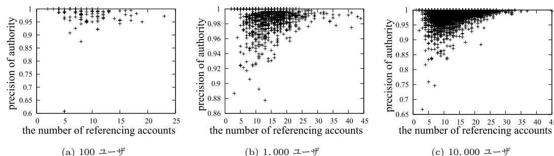
図 6 アクセス権限適合率の分布 Fig. 6 Distribution of users.
