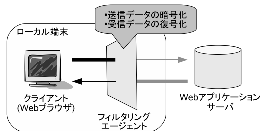
図1 フィルタリング・エージェントシステム Fig.1 Filtering agent system.
