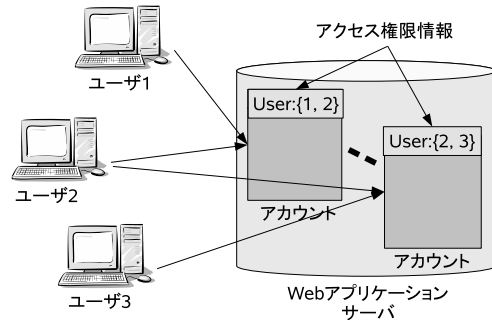
図 4 マルチアカウントモデル Fig. 4 Multi account model.
