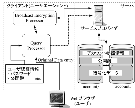
図2 フレームワーク構造とデータの流れ Fig. 2 Framework and dataflow.
