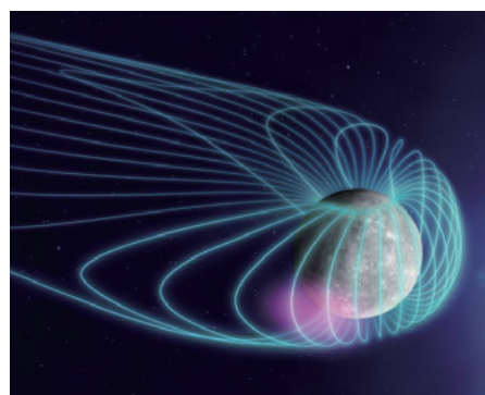
水星でのコーラス波動発生イメージ図 (Credit: 金沢大学、水星画像: NASA/Johns Hopkins University Applied Physics Laboratory/Carnegie Institution of Washington)
