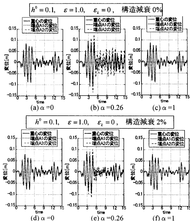
図 4 地震時応答解析結果
