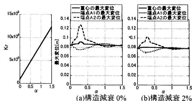
図 5 地震時最大変位応答 ( h^0=0.1 , \epsilon=1.0 , \epsilon_k=0 )
