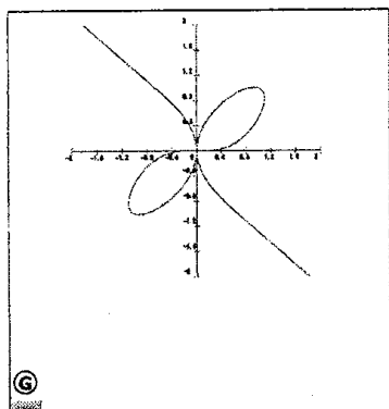
図 6: 一関数グラフ
