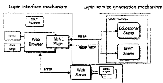
図 15: WME と Lupin の関係
