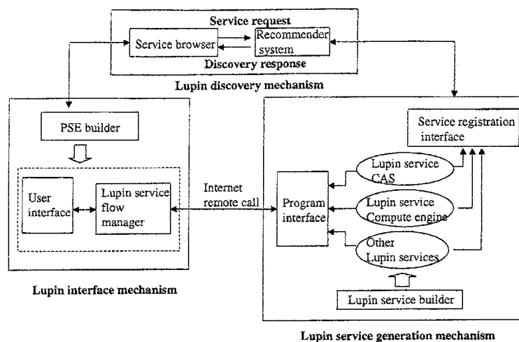
図 1: Lupin のアーキテクチャ
