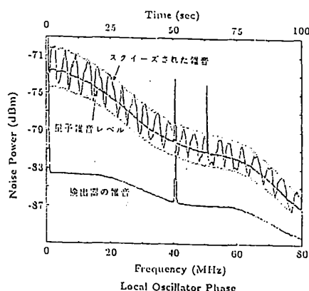
図 3: パルス光によるスクイズド光の発生と観測
