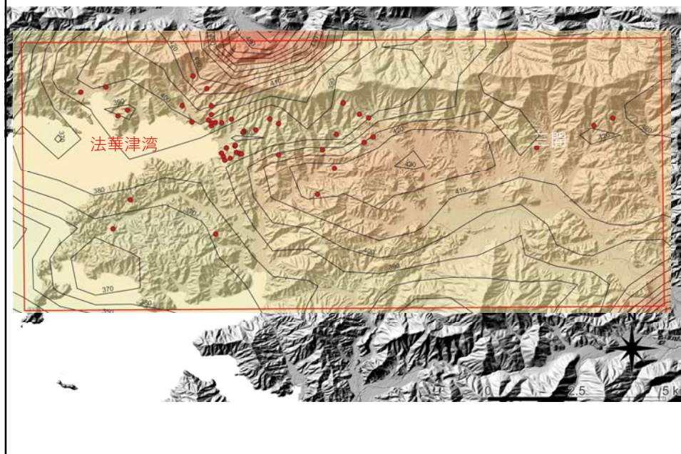
7月5日～7日までの72時間雨量分布＋深さ2 m以上の崩壊（赤丸）
