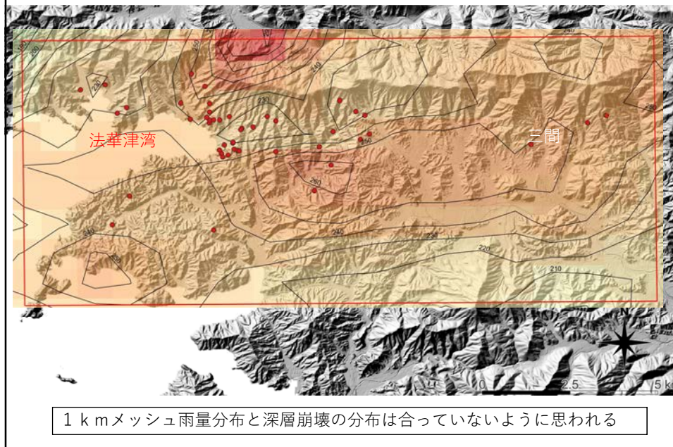
7月7日12時までの12時間雨量分布＋深さ2 m以上の崩壊（赤丸）
