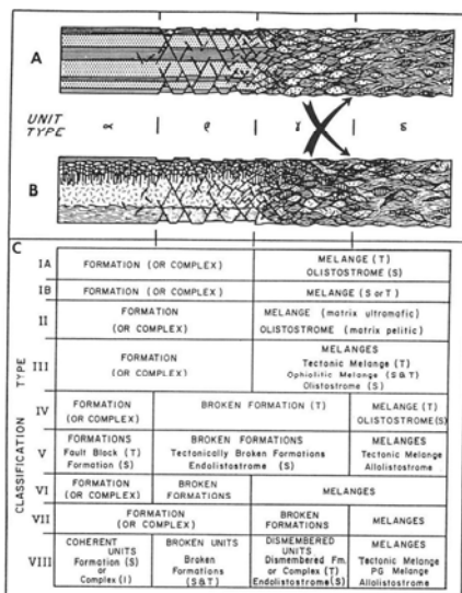
図3-3 メランジュとそれに関係した岩体の特徴と分類 (Raymond, 1984)
