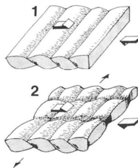
図2-8 層平行剪断(1)に重複した層平行伸張(2)に伴うブーダン化によるメランジュ岩塊の形成モデル (Kimura & Mukai, 1991)
