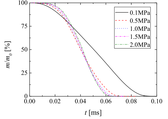
(b) T_0=1500 K (Case 13)
