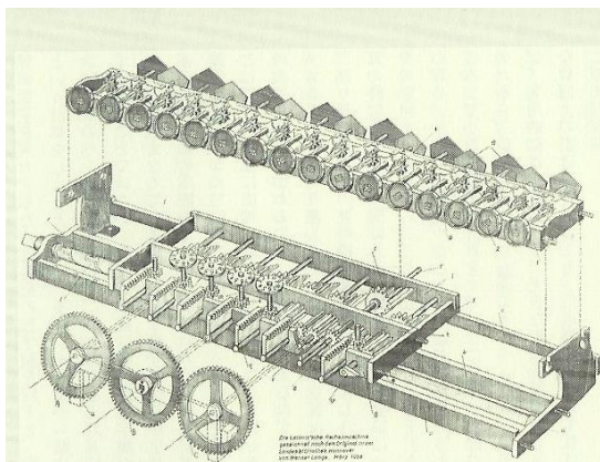
(左図：ライプニッツ考案の計算機の内部構造 右図：段違い歯車の仕組)
