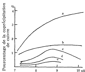
Fig. 2. Variation de la quantité de cuivre coprécipité avec le pH.
