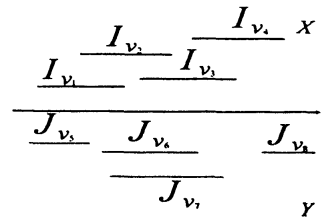
図 4 区間表現
