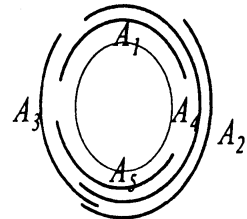
図 7 円弧表現
