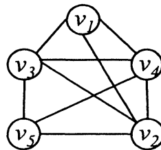
図 6 円弧グラフ
