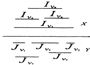
図 2 区間表現
