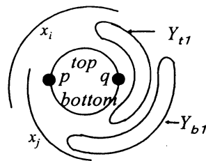
図 14 円弧表現
