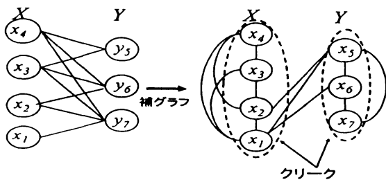
図 10 二部グラフの補グラフの性質についての例
