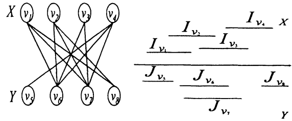
図 3 真区間二部グラフ
