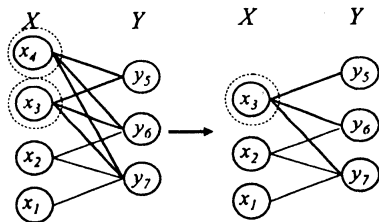
図 13 twin の関係にある頂点集合を一頂点に縮約
