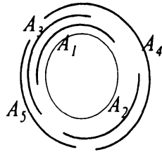
図 9 円弧表現
