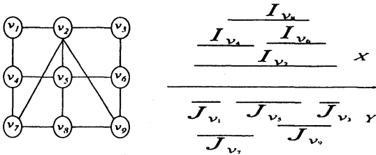
図 1 区間二部グラフ
