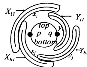
図 15 円弧表現
