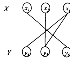
図 11 真区間二部グラフ G
