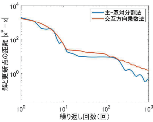
図 1 収束の様子
