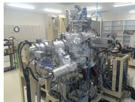
スパッタリング薄膜作製装置
