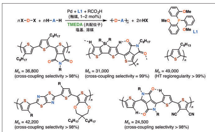
図2 直接的アリール化重合によって合成したπ共役系高分子の例
