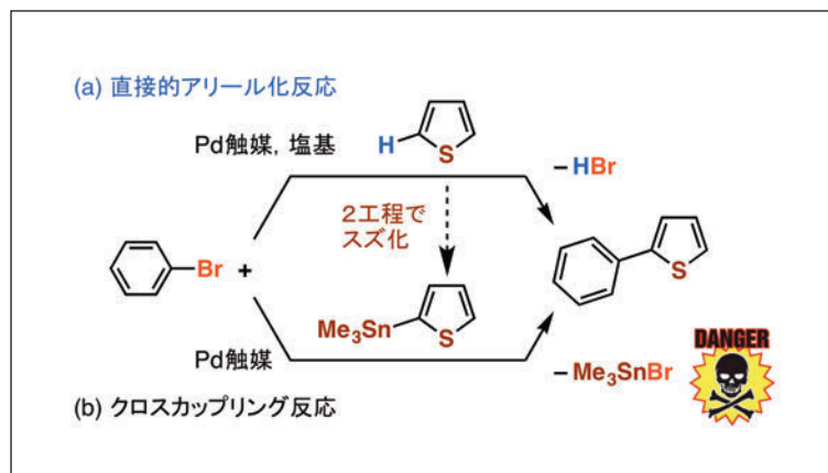
図1 直接的アリール化反応と有機スズ反応剤を用いるクロスカップリング反応との比較。スズ化に伴う反応工程と、毒性の強い有機スズ化合物の副生を回避できる。
