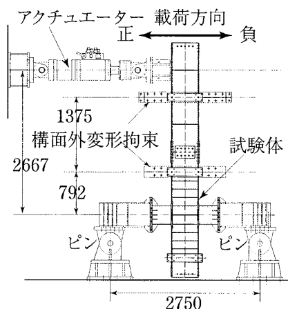
図 1 载荷装置 (単位: mm)
