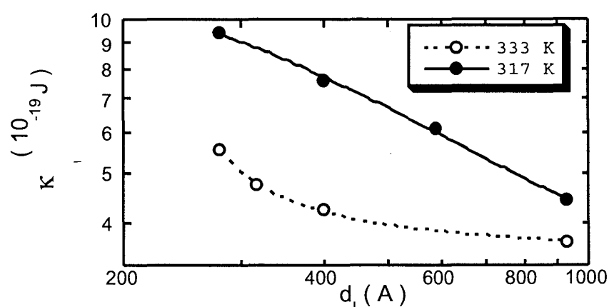
図 2. NSE の解析に Zilman らの理論を用いて得られた DPPC/D 2 O/CaCl 2 系 (CaCl 2 : 7mM) における脂質 2 重層膜の曲げの弾性率 \kappa の膜間隔周期 d への依存性
