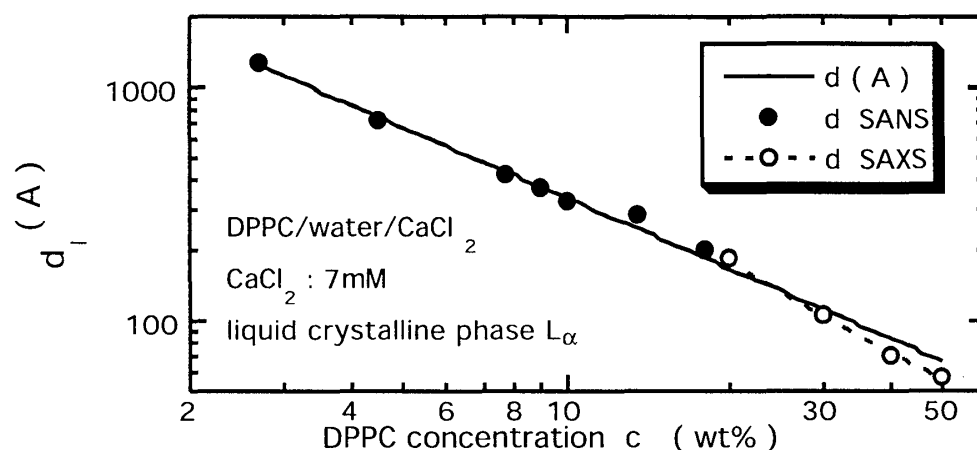
図 1. 回折ピークから得られた膜間隔周期 d の DPPC 濃度 c への依存性。実線は d \propto c^{-1} を示す。
