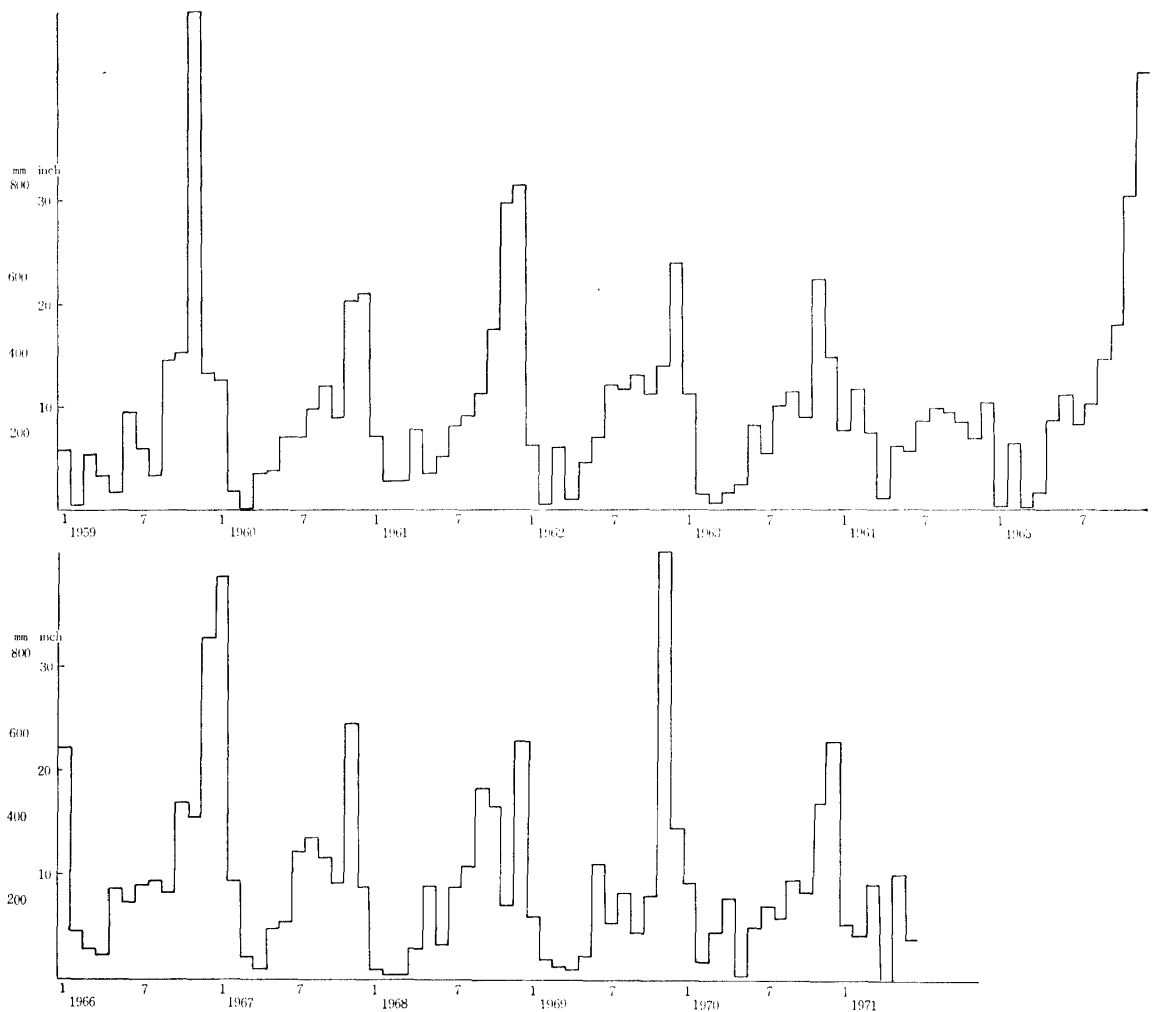
図2 月別雨量 1959.1~1971.6
