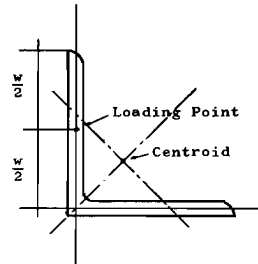
Fig. 18. Web member.
