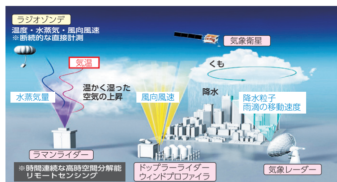
気温・水蒸気ラマンライダーの気象分野における活用イメージ。雲生成前の大気を計測することで、大雨をもたらす雲の発生をより早期に予測できることが期待されています。
