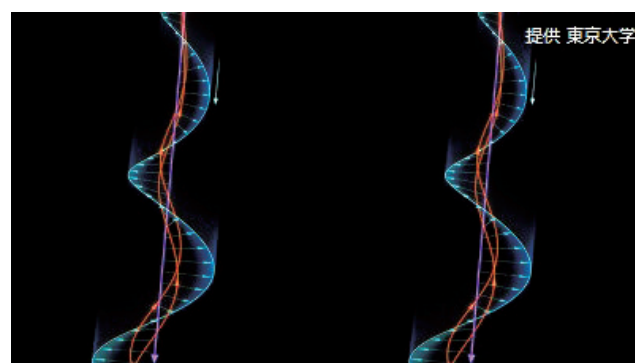
磁場(紫)に沿って伝わる電波(水色)とすれ違う電子(赤)のイメージ。このすれ違う過程で、エネルギーが電子から電波へ受け渡される(提供: 東京大学)
