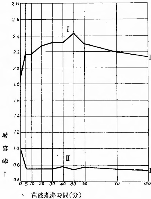
第13表 馬正常血清ヲ以テセルフレキシネル型赤痢菌液煮沸時間ト増容反應(實驗第一七)
