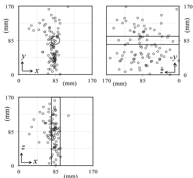
図-3 \text{CO}_2 圧入時の AE 震源分布。左上は水平面（xy 平面）、左下（xz 平面）と右上（yz 平面）は鉛直面に対する AE 震源の投影図。
