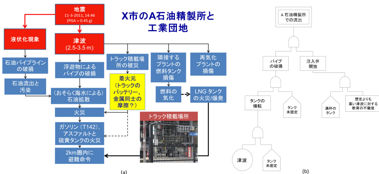
図-4 (a) X 市の工業団地における津波被害を単純化したイベントツリー (b) A 石油精製所において津波をトップイベントとした場合の石油流出のフォルトツリーの抜粋
