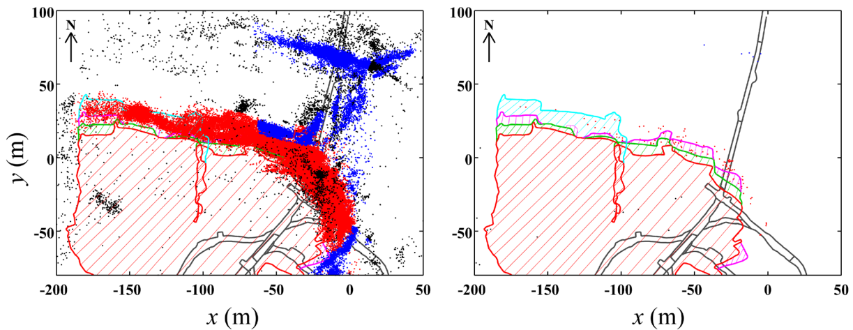
図-4 南アフリカのある金鉱山の地下 1km に展開した観測網で検知された微小破壊の震源分布（平面図）。左）検知された全イベント。小さいものでは M - 5 以下のイベントが検知できている。図左下の斜線部は鉱脈の採掘跡を表す。右）左図に示した震源のうち、 M - 1 以上（鉱山に展開される典型的な地震観測網で検知できる規模のイベント）のみをプロットしたもの。左の図では、様々な場所に集中する微小破壊がはっきりと確認できるが、右の図ではほとんど何もわからない。
