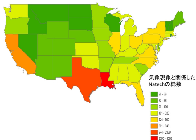
図-2 アメリカ合衆国で 1990 - 2008 年の間に起きた気象現象と関係した Natech 事故 (NRC からデータを引用)
