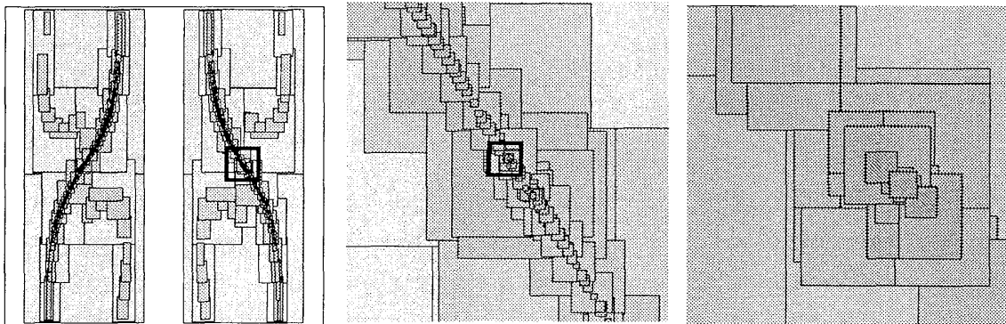
図 14: レベル生成の一例: 15 段のレベルを積んだ状態。図中の太線で囲われた領域を拡大して表示している。強いフロントが形成されている所に細かいメッシュが集中している。
