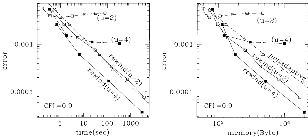
図 10: SOD 問題における、メモリーおよび計算時間と誤差の関係。左下側にいくほど効率がよい計算であることを示している。誤差は L^2 ノルムで評価した。白い三角形は、AMR 法を用いない通常のメッシュ計算で、メッシュ数は 800, 1600, 3200, 6400, 12800, 25600 である。nonadaptive と書いた一点鎖線は、best fit の直線である。四角で書いたものは、AMR 計算によるものである。実線は、rewind を行った場合、破線は rewind を用いなかった場合である。 u の値は、upper level factor である。白い四角形は u = 2 の場合、黒い四角形は u = 4 の場合にそれぞれ相当する。格子数は、level \ell = 0 のメッシュで 100、 \ell_{\max} は u = 2 の場合が 3, 4, 5, 6, 7, 8, 9、 u = 4 の場合が 2, 3, 4, 5 である。
