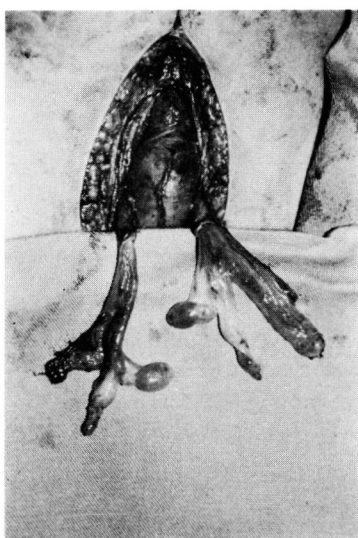
Fig. 3. 手術所見
