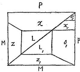
第一四圖 バベノ式双晶
