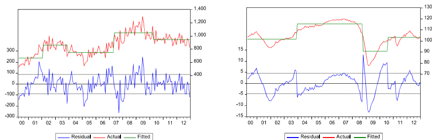
(図8) 企業倒産件数のレジーム分割(左)と Composite Index のレジーム分割(右)
