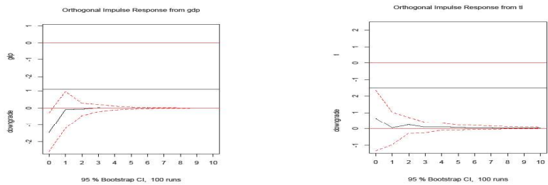
(a) GDP →「過去の信用イベントの影響+frailty」 (b) 総与信額 → 「過去の信用イベントの影響+frailty」
