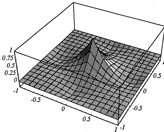
図 6: node が \hat{\Omega}_k の頂点にある場合
