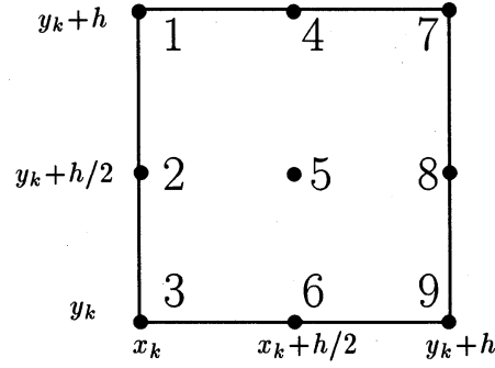
図 5: element node numbers
