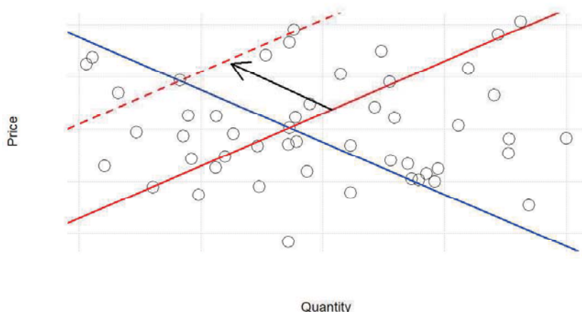
Figure 8: 需要曲線（blue）と内向きにシフトする供給曲線（red）を重ね合わせた模擬数量に対する模擬均衡価格の散布図
