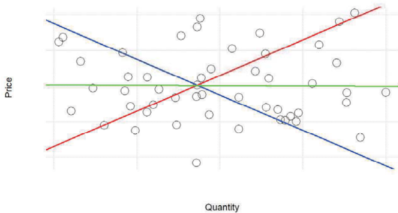
Figure 5: 需要曲線 (blue) と供給曲線 (red) と推定回帰直線 (green) を書き込んだ模擬均衡数量に対する模擬均衡価格の散布図
