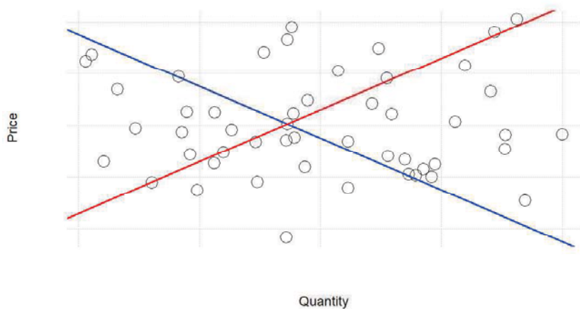
Figure 4: 需要曲線 (blue) と供給曲線 (red) を書き込んだ模擬均衡数量に対する模擬均衡価格の散布図
