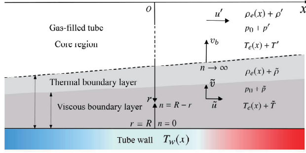
図 1: 壁面温度が軸方向に一樣でない円形断面の管路中の気体内の音場。音場は壁面付近の境界層（拡大され描かれている）とその外部のコア領域とに分けられる。境界層は粘性境界層と温度境界層からなり、壁面に温度勾配があると温度境界層に粘性境界層が影響する。壁面温度 T_w が軸 x 方向に緩やかに変化しているときには、静止状態（一樣な圧力を p_0 とする）の気体の温度 T_e は断面内で一樣であり、 T_w に等しくおける。記号 (\cdot) と (\cdot)' はそれぞれ境界層およびコア領域での密度、温度、圧力および速度の静止状態での値からの攪乱を表す。
