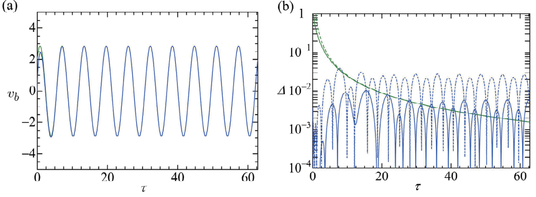
図 3: 境界層外縁速度 v_b の解析解 (3.15) と数値解 (4.22) ( N = 16 ) との比較を (a) に示す. 赤で示す解析解は青の数値解の後ろにあり全く見えない. なお, 係数 \sqrt{\nu_e a_0/L} は省かれている. 緑の線は定常応答 (C + C_T) \cos(\tau - \pi/4) を表す. 解析解と数値解の差の絶対値 \Delta を (b) に示す. 青の実線は N = 16 の場合であり, 破線は N = 8 の場合である. 緑の実線は定常応答との差を示し, 破線は (3.15) の第 2 項目の \tau^{-3/2} の減衰を表す.
