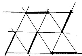
図2. \text{singlet} ペアの作り方のひとつ
