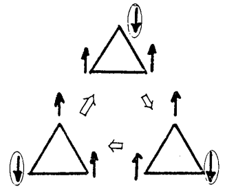
図5. 3角格子上での変換
