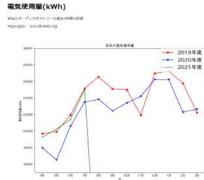
図2 電力使用量のグラフ
