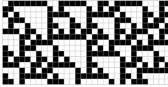
Figure 10. ルール 60 の時間発展の様子
