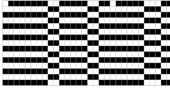
Figure 6. ルール 19 の時間発展の様子
