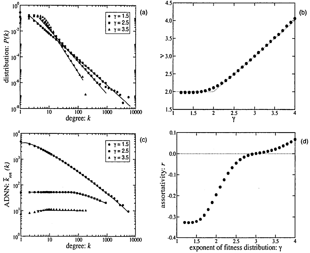
図 1: (a) 結合度分布の例。実線は解析的な計算によって求めた予想 (27), (28) による。 (b) 内的結合強度 a の分布の冪指数 \gamma に対するネットワークの次数分布の冪指数 \nu の変化。黒丸は数値計算の結果であり, m = 3 , d = 2 , N = 10000 の場合である。この結果は d にはよらない。 (c) 次数相関の例。実線は解析的な計算によって求めた予想 (29), (30), (31) による。 (d) 内的結合強度 a の分布の冪指数 \gamma に対する同類度 (assortativity) の変化。 \gamma = 3 を境に正負が入れ替わる。
